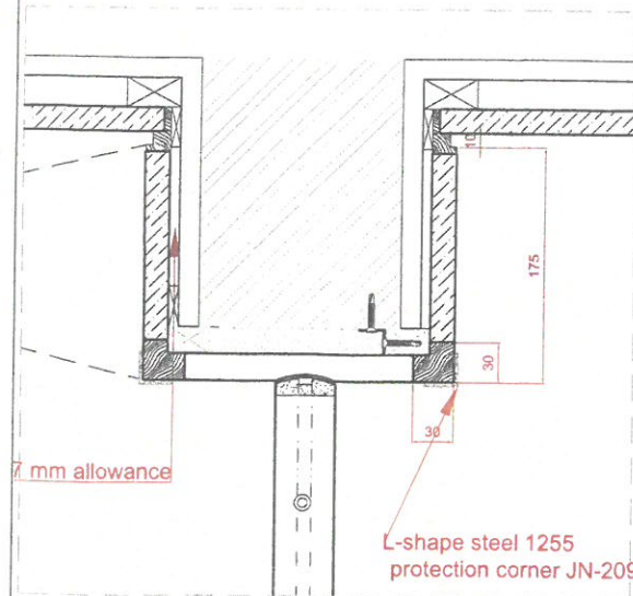
D1 Junction details
